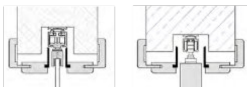
Deckenmontage im Sturz
