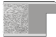
Türblatt Rund-Postformingkante (RP) ca. 5,5 mm Radius
