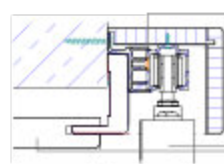
Montage mit Schiebetürfutter für Holztür
