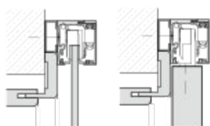
Montage mit DUFU mit Distanzprofil
