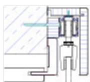
Montage mit Schiebetürfutter für Glastür
